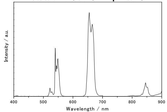
発光スペクトル (1.06 \mu m励起)
